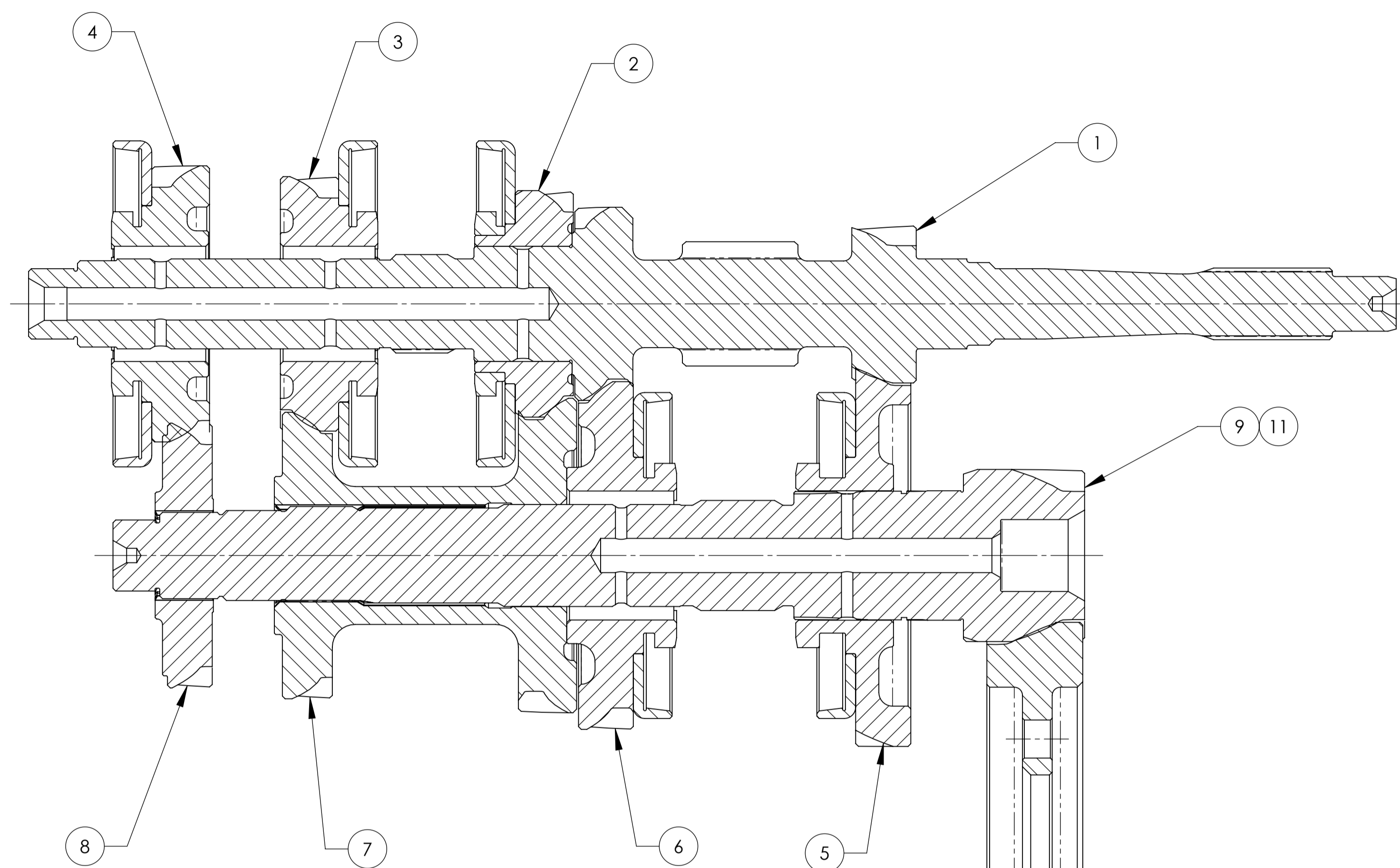
SECTION A-A
